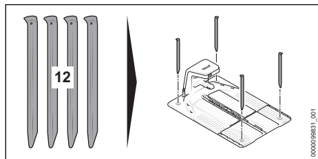
12 Грунтовой гвоздь Четыре грунтовых гвоздя соединяют док-станцию с грунтом.
